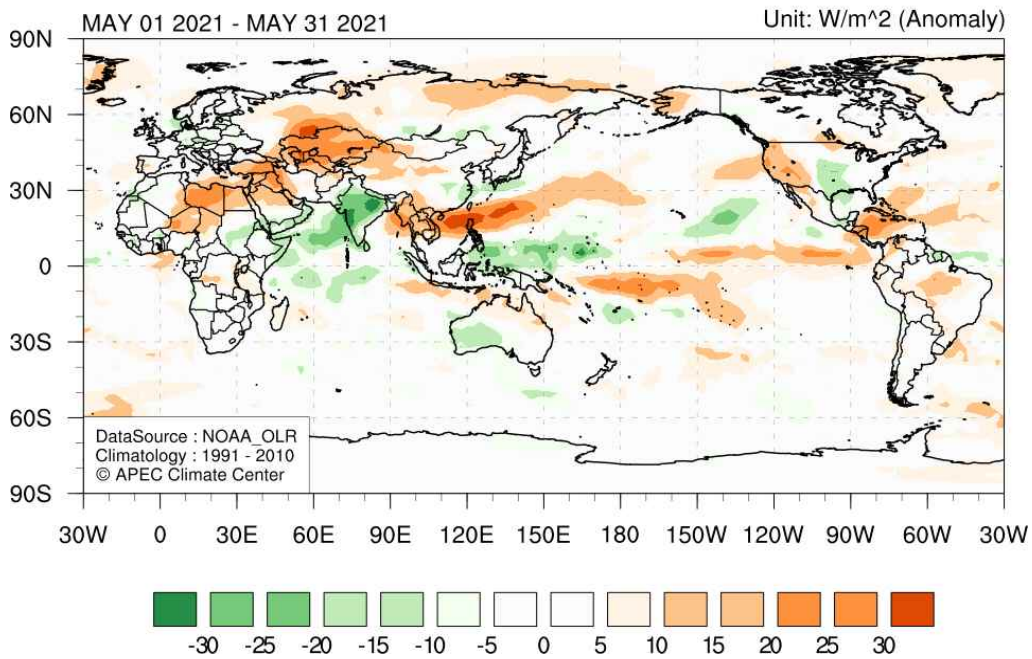
그림 4. (위) 2021년 5월 평균 기온 및 (아래) 상향장파 복사 평년대비 편차 (평년: 1991-2010).
