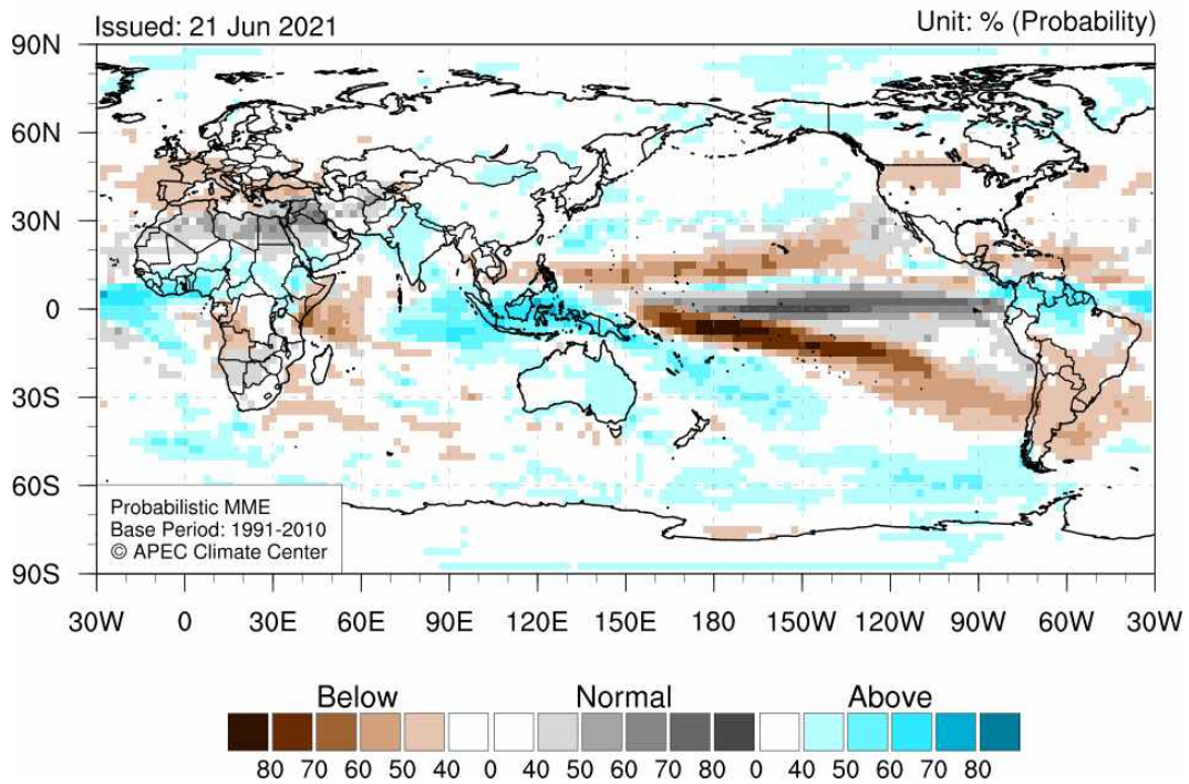
그림 9. (위) 2021년 7월-9월 평균 기온 및 (아래) 강수 평년대비 편차 (평년: 1991-2010).
