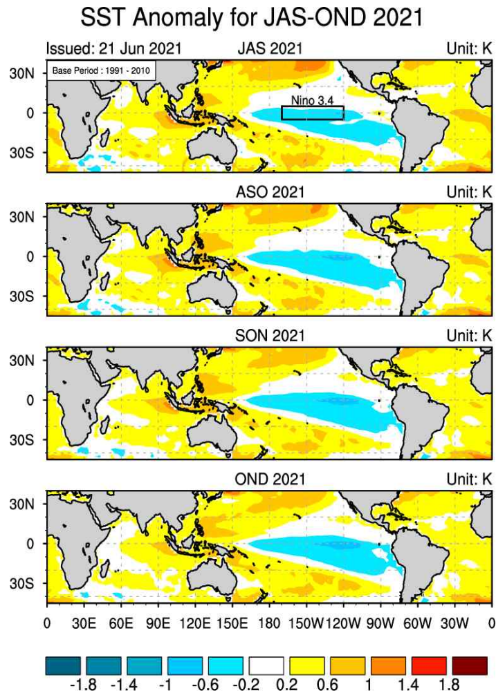
그림 6. 2021년 7월-12월 평균 해수면온도 평년대비 편차 (평년: 1991-2010).
