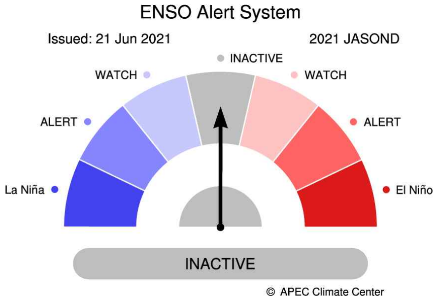
그림 5. 2021년 7월-12월 ENSO 경보 (평년: 1991-2010).
