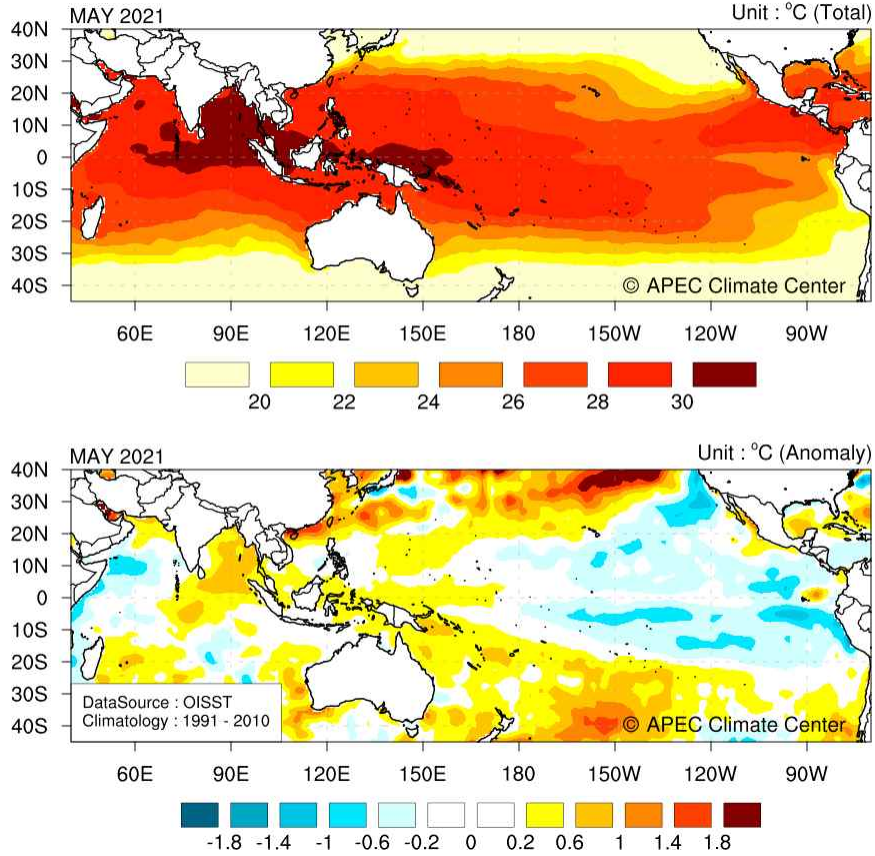
그림 2. 2021년 5월 평균 해수면온도 분포 및 평년대비 편차.
