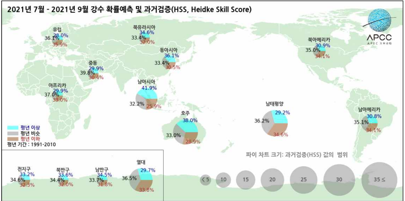
그림 1. (위) 2021년 7월-9월 평균 기온 및 (아래) 강수 확률예측 및 과거검증.
