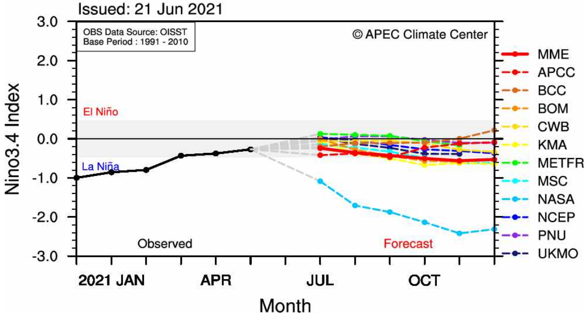
그림 7. 2021년 7월-12월 평년대비 Niño3.4 지수 편차 (평년: 1991-2010).
