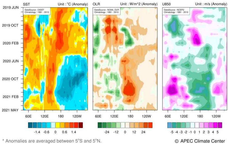
그림 3. 2019년 6월-2021년 5월 해수면온도, 상향장파 복사, 850hPa 바람 평년대비 편차의 시간-경도 단면도 (평년: 1991-2010).
