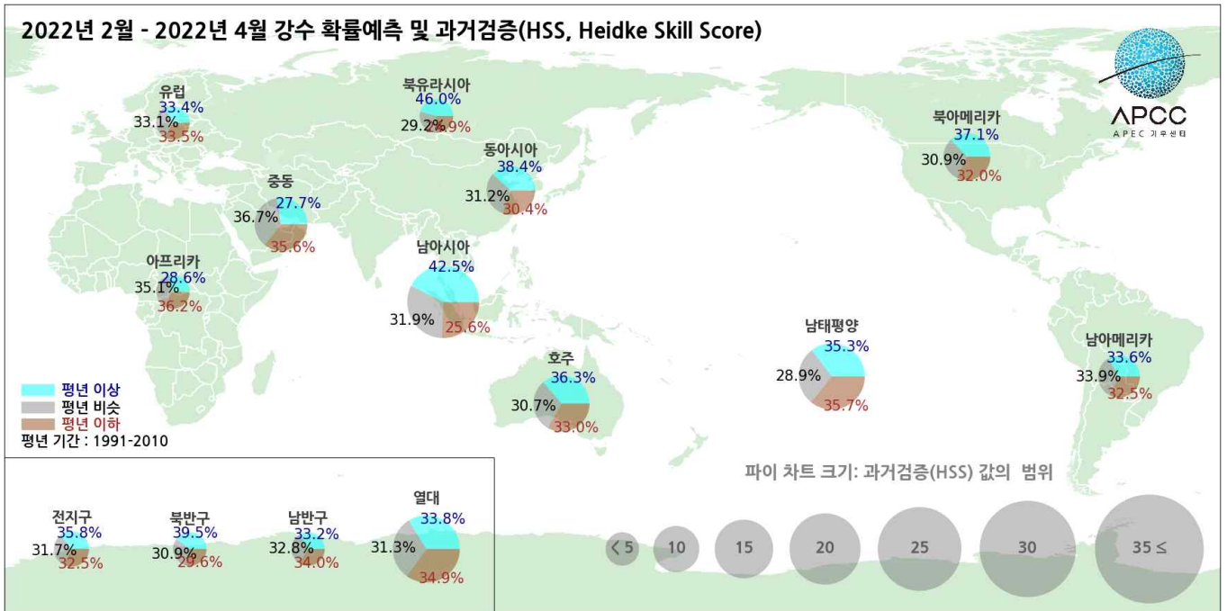
그림 1. 2022년 2월-4월 기온(위)과 강수(아래)의 확률예측 및 과거검증.
