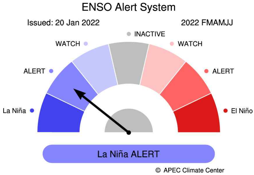
그림 5. 2022년 2월-7월 ENSO 경보(평년: 1991-2010).
