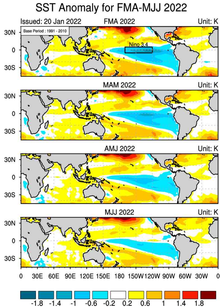
그림 6. 2022년 2월-7월 해수면온도 평년대비 편차(평년: 1991-2010).
