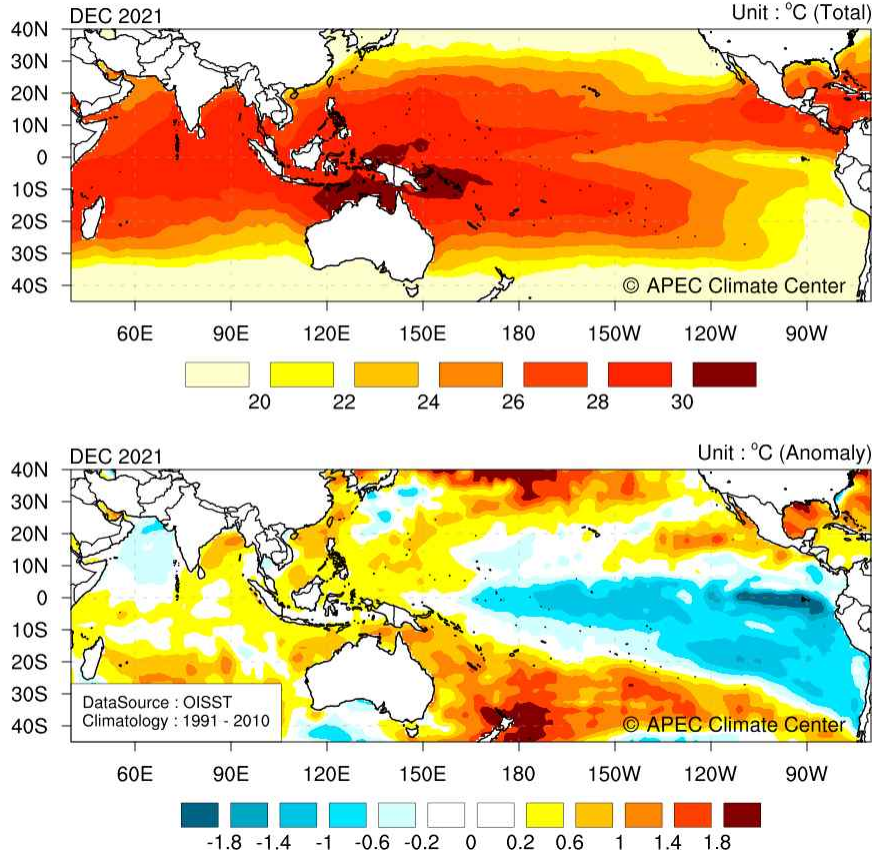
그림 2. 2021년 12월 해수면온도 분포 및 평년대비 편차.
