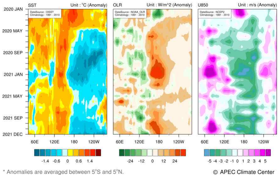
그림 3. 2020년 1월-2021년 12월 해수면온도, 상향장파 복사, 850hPa 바람 평년대비 편차의 시간-경도 단면도(평년: 1991-2010).
