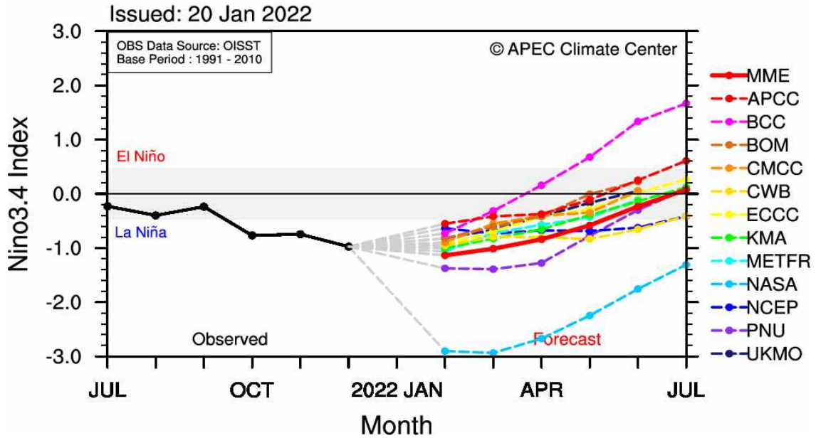
그림 7. 2022년 2월-7월 평년대비 Niño3.4 지수 편차(평년: 1991-2010).
