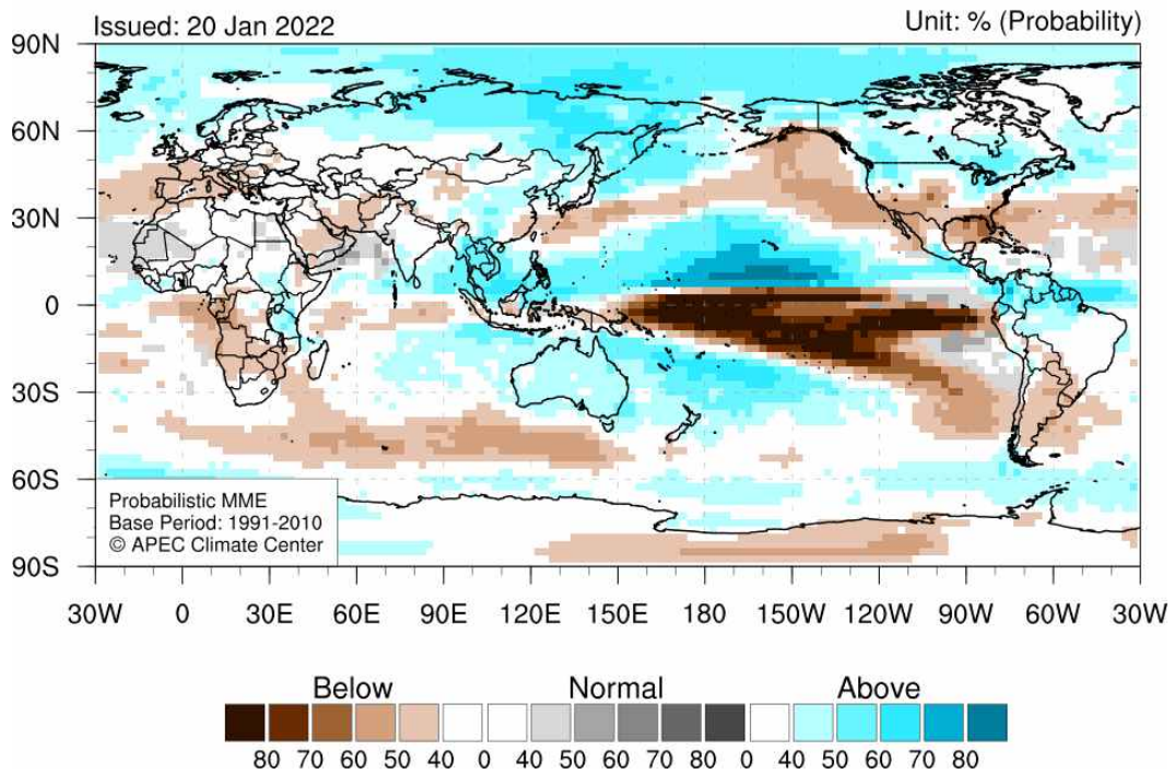
그림 9. 2022년 2월-4월 기온(위)과 강수(아래)의 평년대비 편차(평년: 1991-2010).
