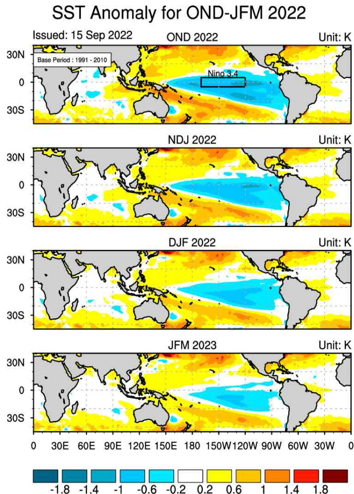
그림 6. 2022년 10월-2023년 3월 해수면온도 평년대비 편차(평년: 1991-2010).
