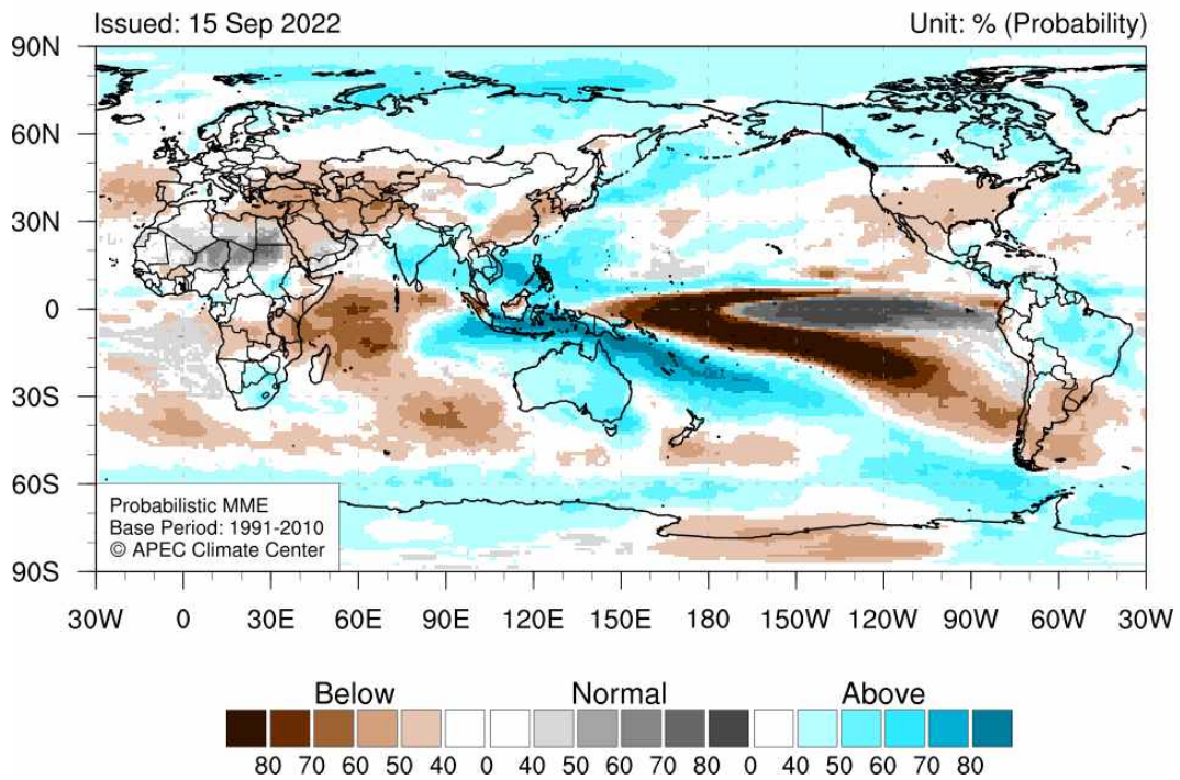
그림 9. 2022년 10월-12월 기온(위)과 강수(아래)의 평년대비 편차(평년: 1991-2010).
