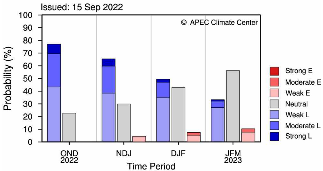
그림 8. 2022년 10월-2023년 3월 ENSO 종류 및 강도 확률예측(평년: 1991-2010).
