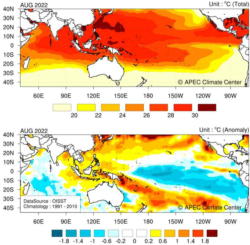
그림 2. 2022년 8월 해수면온도 분포 및 평년대비 편차.
