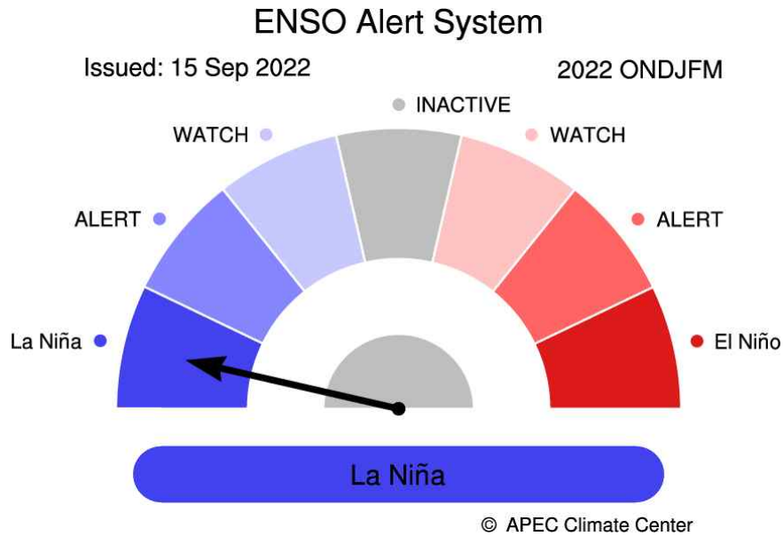
그림 5. 2022년 10월-2023년 3월 ENSO 경보(평년: 1991-2010).
