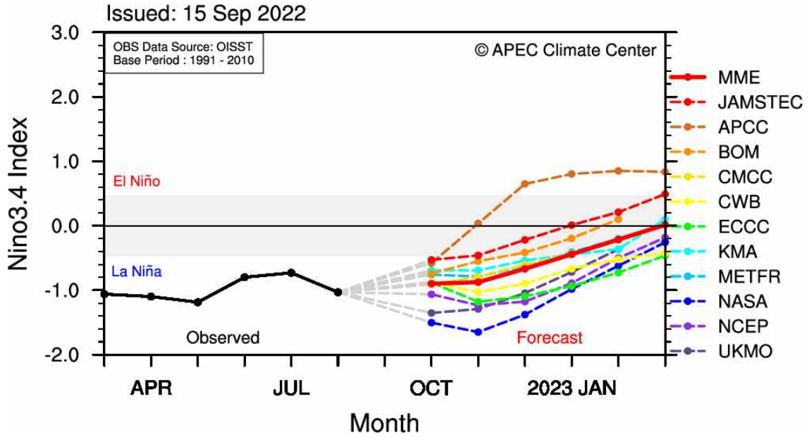
그림 7. 2022년 10월-2023년 3월 평년대비 Niño3.4 지수 편차(평년: 1991-2010).
