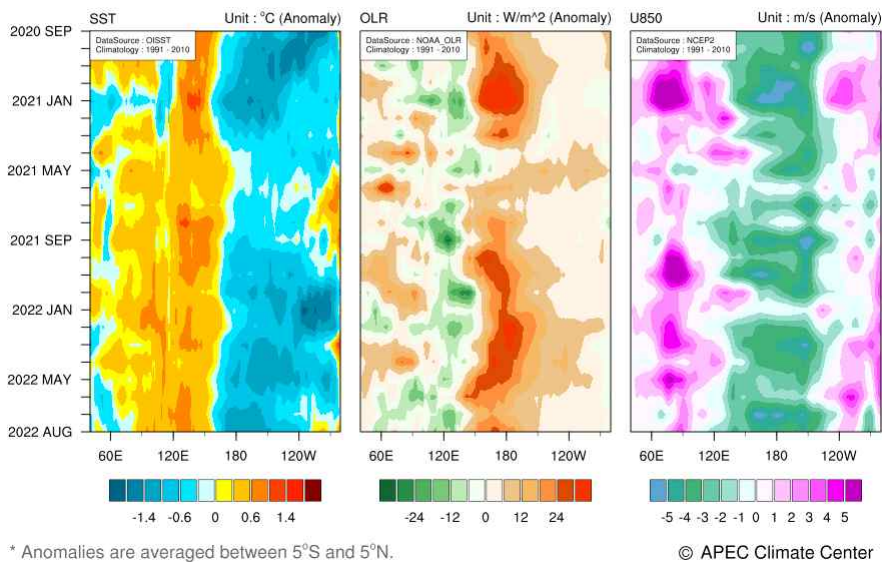
그림 3. 2020년 9월-2022년 8월 해수면온도, 상향장파복사, 850hPa 바람 평년대비 편차의 시간-경도 단면도(평년: 1991-2010).
