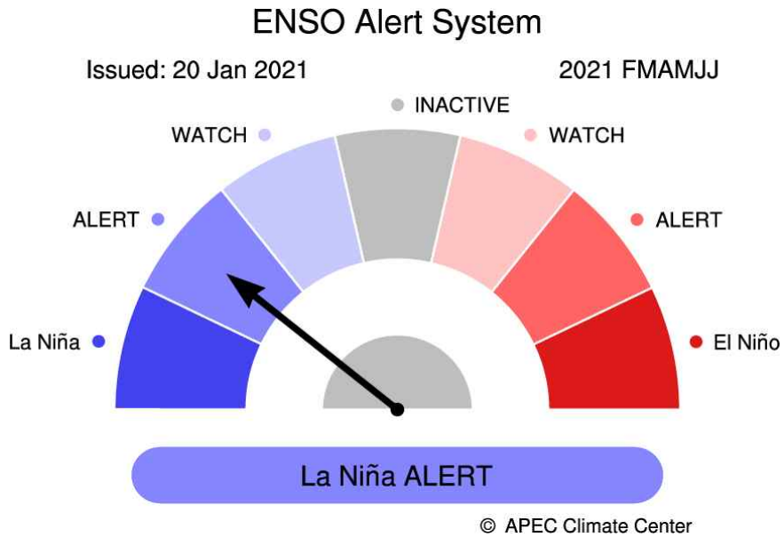
그림 5. 2021년 2월-7월 ENSO 경보 (평년: 1991-2010).
