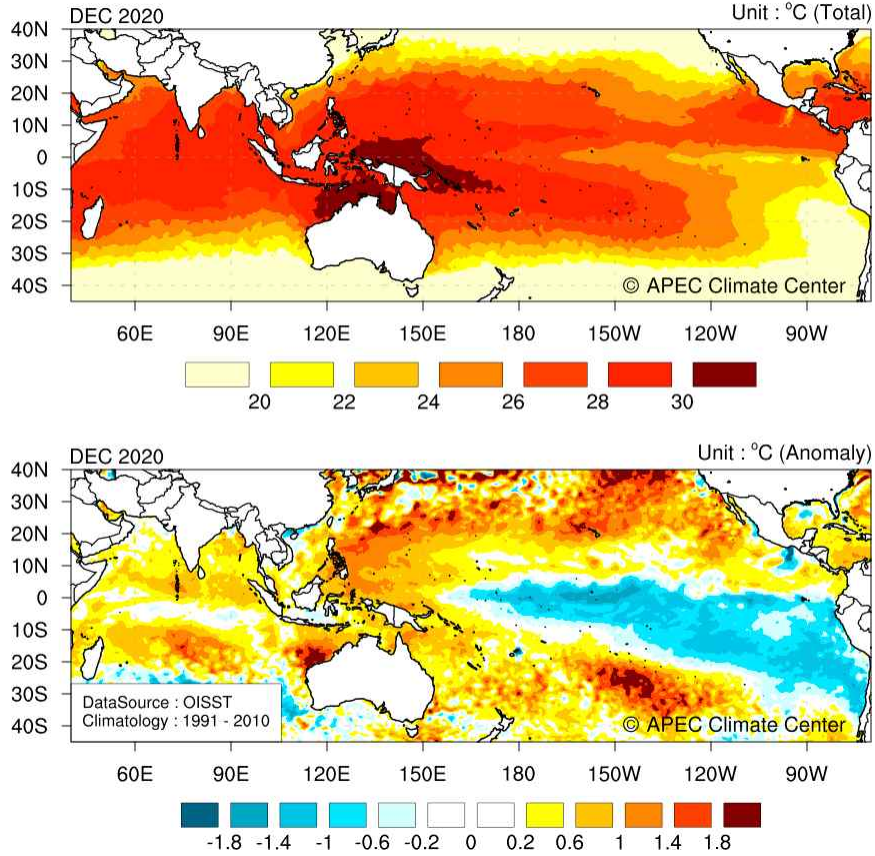
그림 2. 2020년 12월 평균 해수면온도 분포 및 평년대비 편차.
