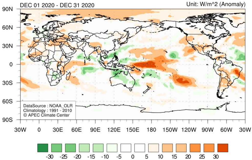
그림 4. (위) 2020년 12월 평균 기온 및 (아래) 상향장파 복사 평년대비 편차 (평년: 1991-2010).
