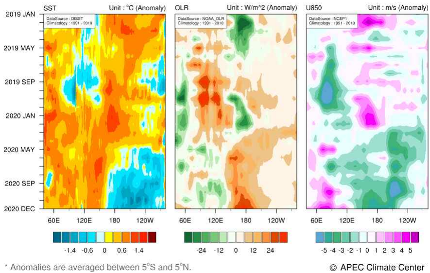
그림 3. 2019년 1월-2020년 12월 해수면온도, 상향장파 복사, 850hPa 바람 평년대비 편차의 시간-경도 단면도 (평년: 1991-2010).
