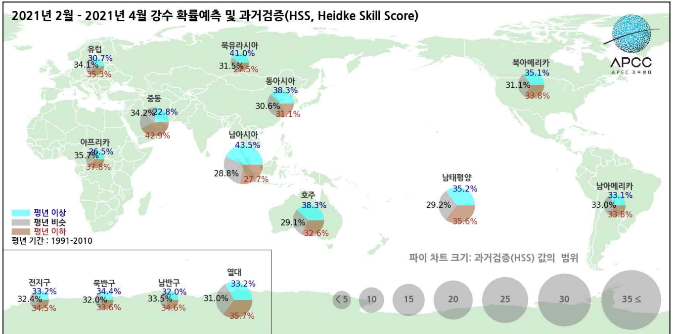
그림 1. (위) 2021년 2월-4월 평균 기온 및 (아래) 강수 확률예측 및 과거검증.
