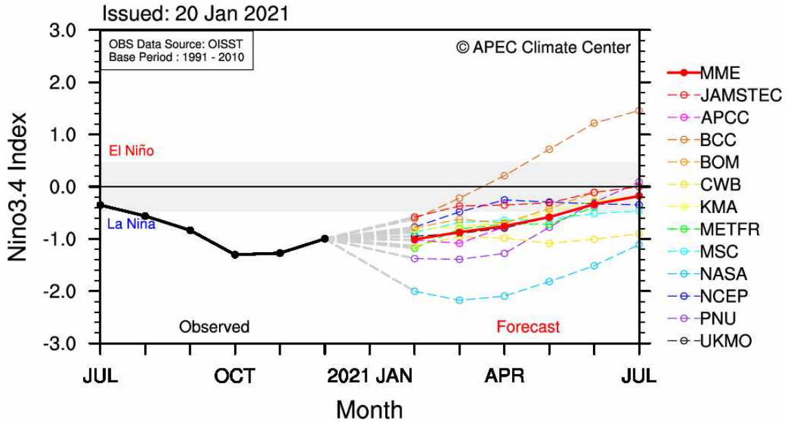
그림 7. 2021년 2월-7월 평년대비 Niño3.4 지수 편차 (평년: 1991-2010).
