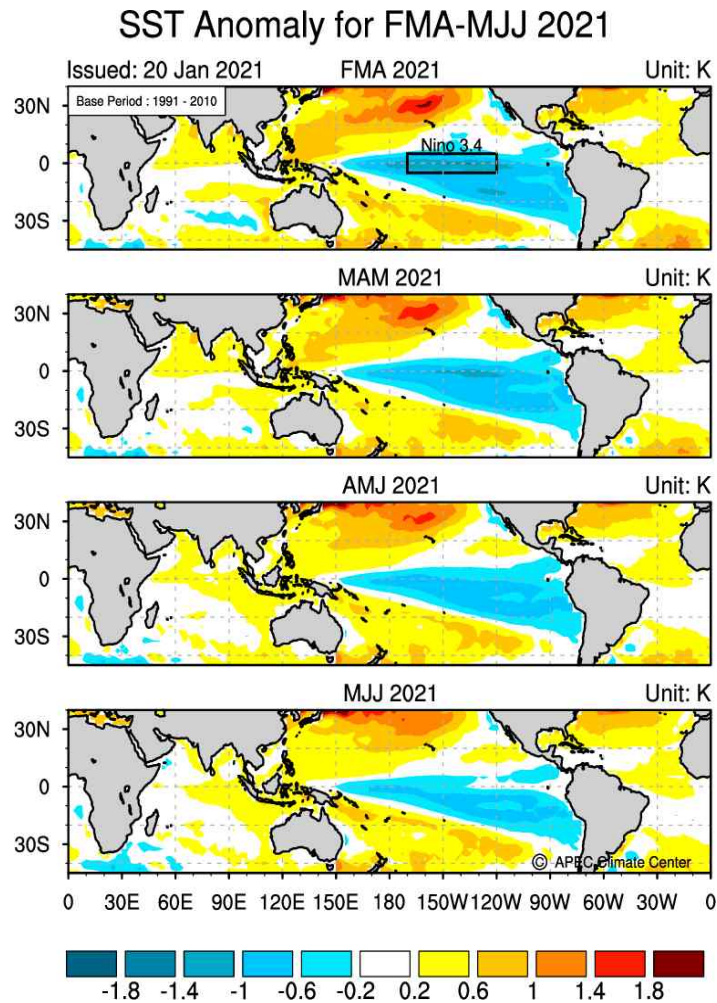
그림 6. 2021년 2월-7월 평균 해수면온도 평년대비 편차 (평년: 1991-2010).
