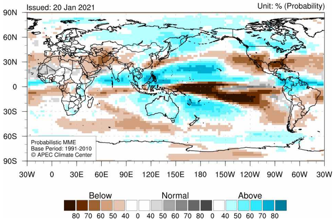
그림 9. (위) 2021년 2월-4월 평균 기온 및 (아래) 강수 평년대비 편차 (평년: 1991-2010).
