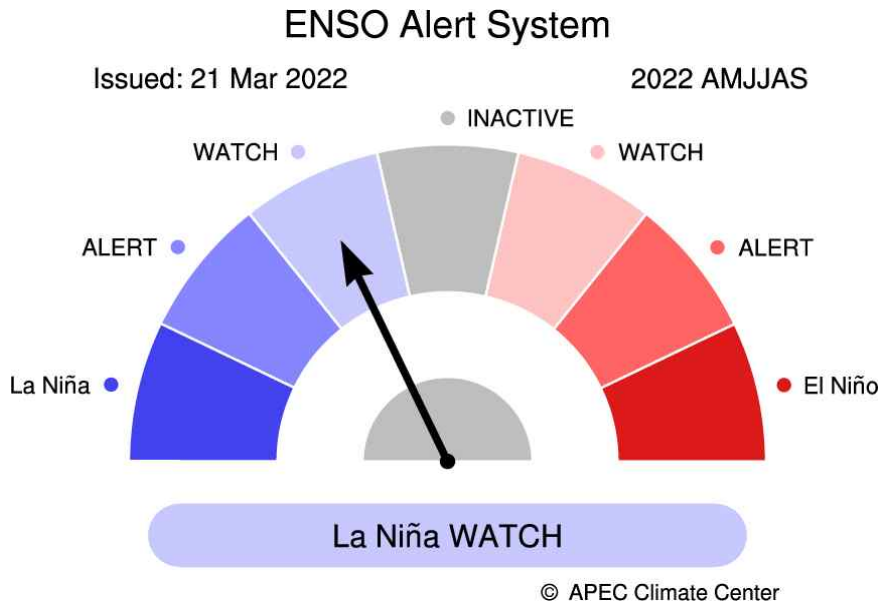
그림 5. 2022년 4월-9월 ENSO 경보(평년: 1991-2010).
