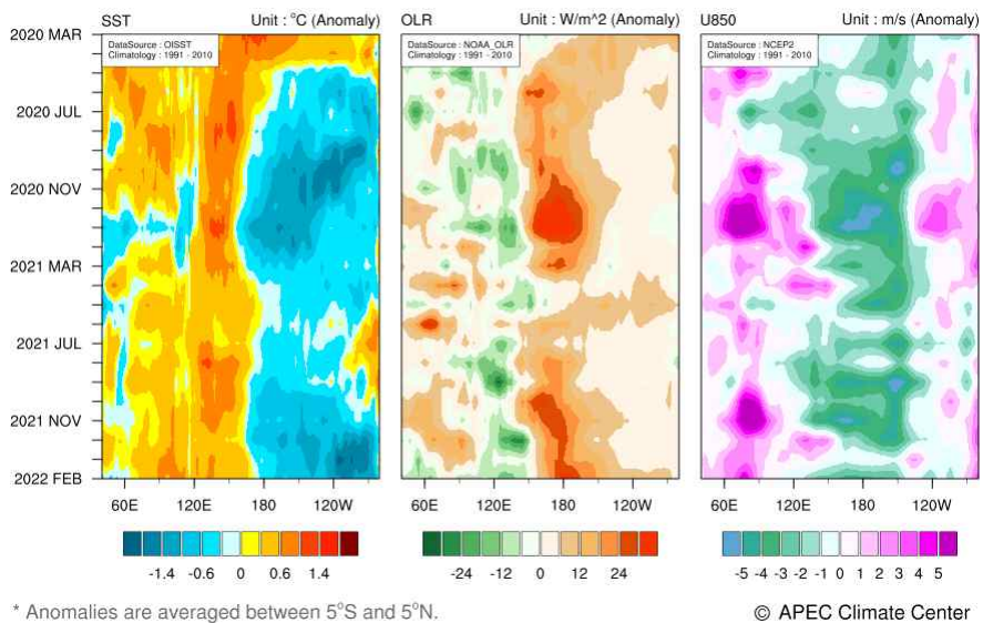
그림 3. 2020년 3월-2022년 2월 해수면온도, 상향장파복사, 850hPa 바람 평년대비 편차의 시간-경도 단면도(평년: 1991-2010).
