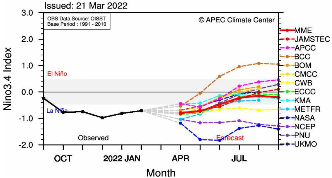
그림 7. 2022년 4월-9월 평년대비 Niño3.4 지수 편차(평년: 1991-2010).
