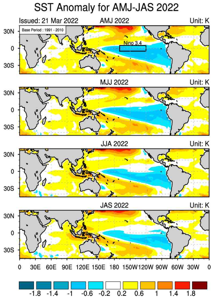
그림 6. 2022년 4월-9월 해수면온도 평년대비 편차(평년: 1991-2010).
