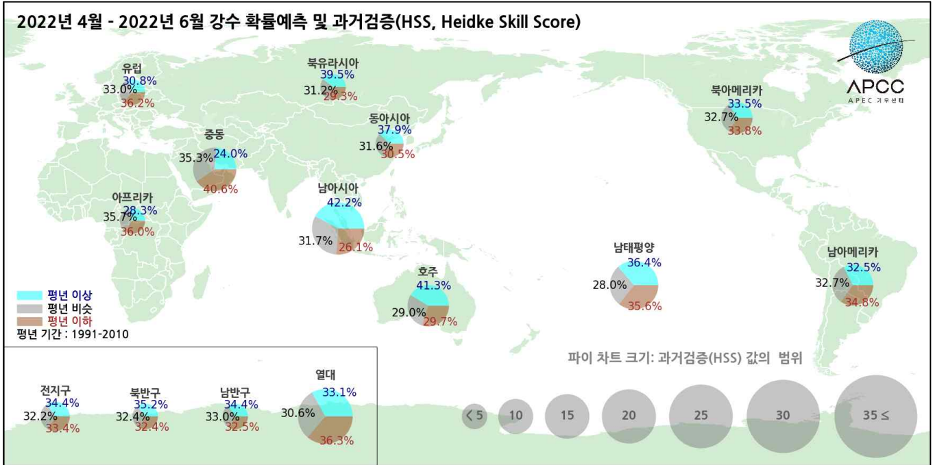
그림 1. 2022년 4월-6월 기온(위)과 강수(아래)의 확률예측 및 과거검증.
