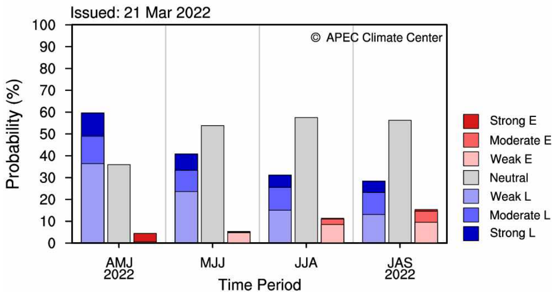
그림 8. 2022년 4월-9월 ENSO 종류 및 강도 확률예측(평년: 1991-2010).
