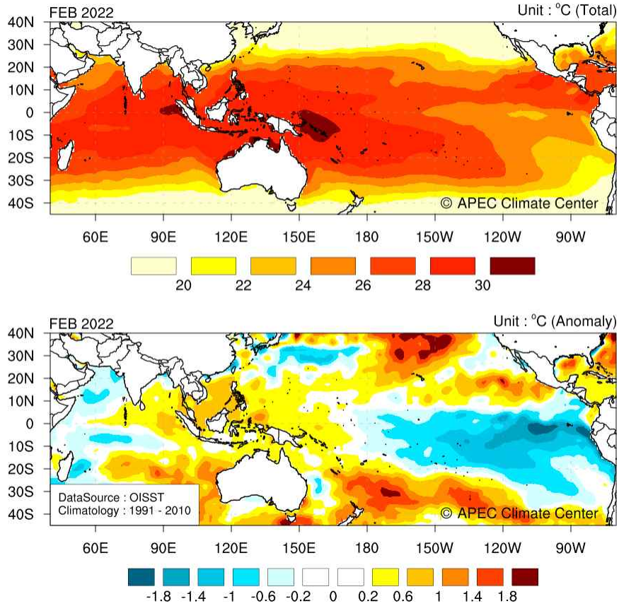
그림 2. 2022년 2월 해수면온도 분포 및 평년대비 편차.
