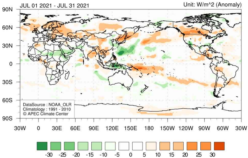
그림 4. (위) 2021년 7월 평균 기온 및 (아래) 상향장파 복사 평년대비 편차 (평년: 1991-2010).
