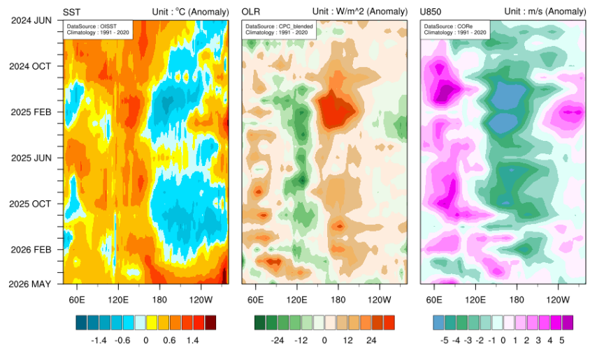
2024 6월 - 2026 5월 적도지역 해수면온도, 상향장파복사, 850hPa 동서 바람 평년대비 편차의 시간-경도 단면도 (평년: 1991- 2020)
