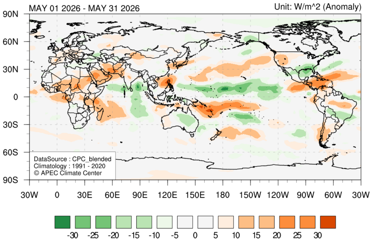
2026 5월 기온 (위) 및 상향장파복사(아래)의 평년대비 편차 (평년 : 1991-2020)
