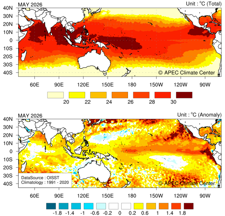
2026 5월 해수면 온도 분포(위) 및 평년대비 편차(아래) (평년: 1991-2020)
