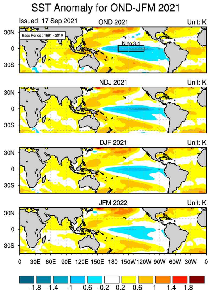
그림 6. 2021년 10월-2022년 3월 평균 해수면온도 평년대비 편차 (평년: 1991-2010).
