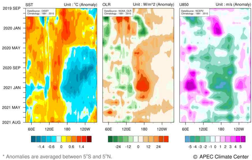
그림 3. 2019년 9월-2021년 8월 해수면온도, 상향장파 복사, 850hPa 바람 평년대비 편차의 시간-경도 단면도 (평년: 1991-2010).
