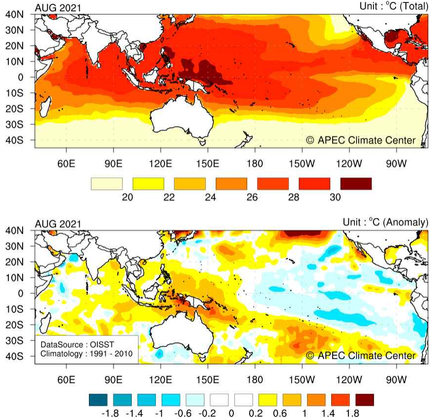
그림 2. 2021년 8월 평균 해수면온도 분포 및 평년대비 편차.
