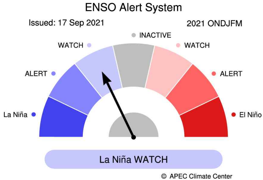
그림 5. 2021년 10월-2022년 3월 ENSO 경보 (평년: 1991-2010).
