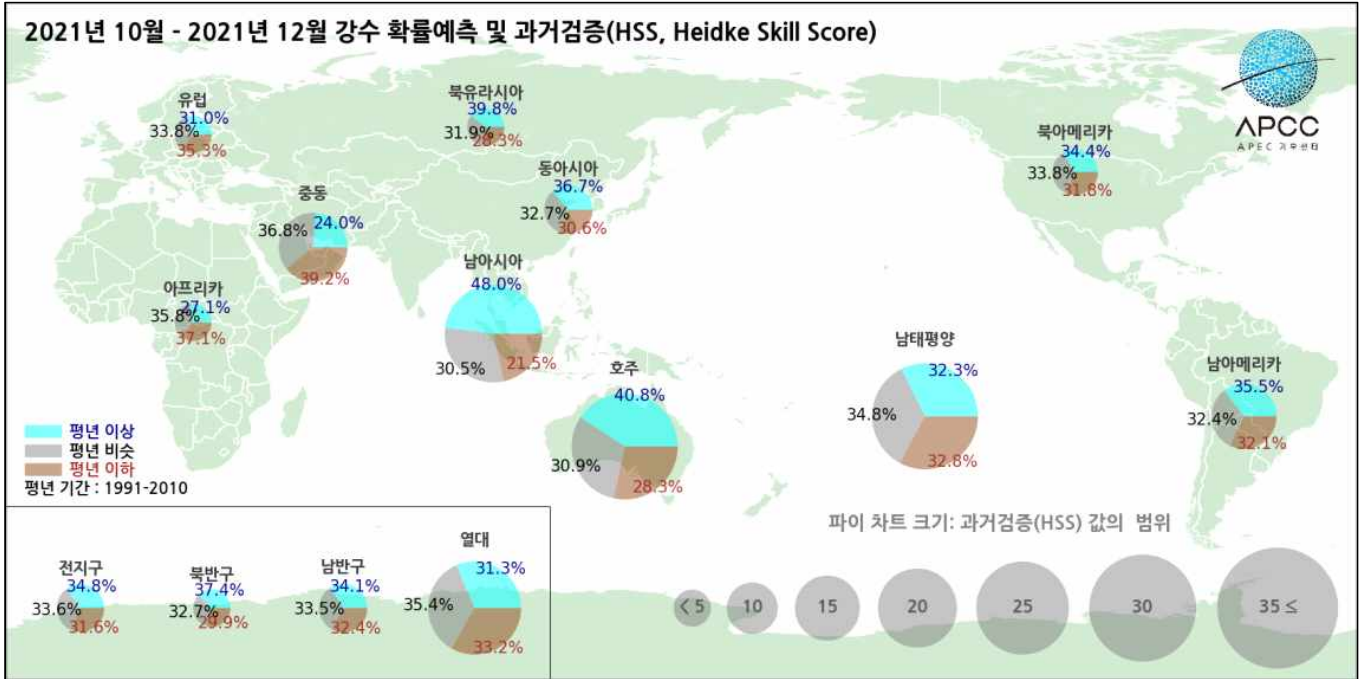
그림 1. (위) 2021년 10월-12월 평균 기온 및 (아래) 강수 확률예측 및 과거검증.
