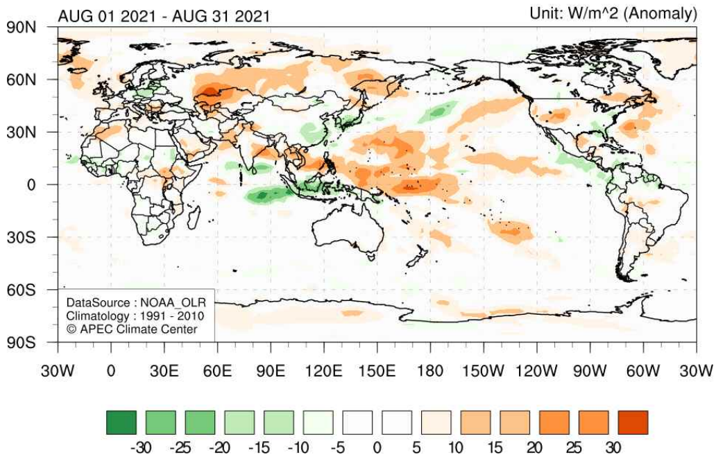
그림 4. (위) 2021년 8월 평균 기온 및 (아래) 상향장파 복사 평년대비 편차 (평년: 1991-2010).
