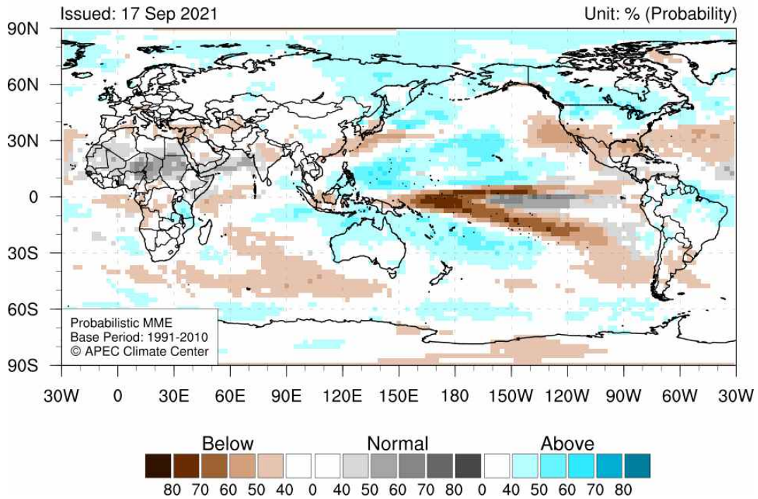
그림 10. (위) 2022년 1월-3월 평균 기온 및 (아래) 강수 평년대비 편차 (평년: 1991-2010).
