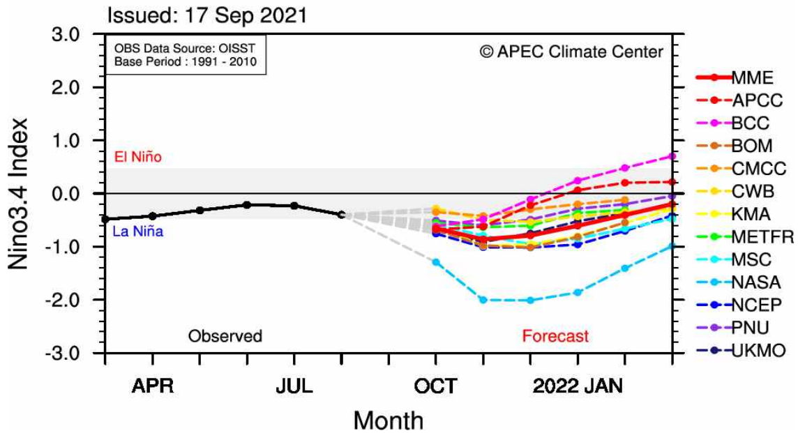
그림 7. 2021년 10월-2022년 3월 평년대비 Niño3.4 지수 편차 (평년: 1991-2010).
