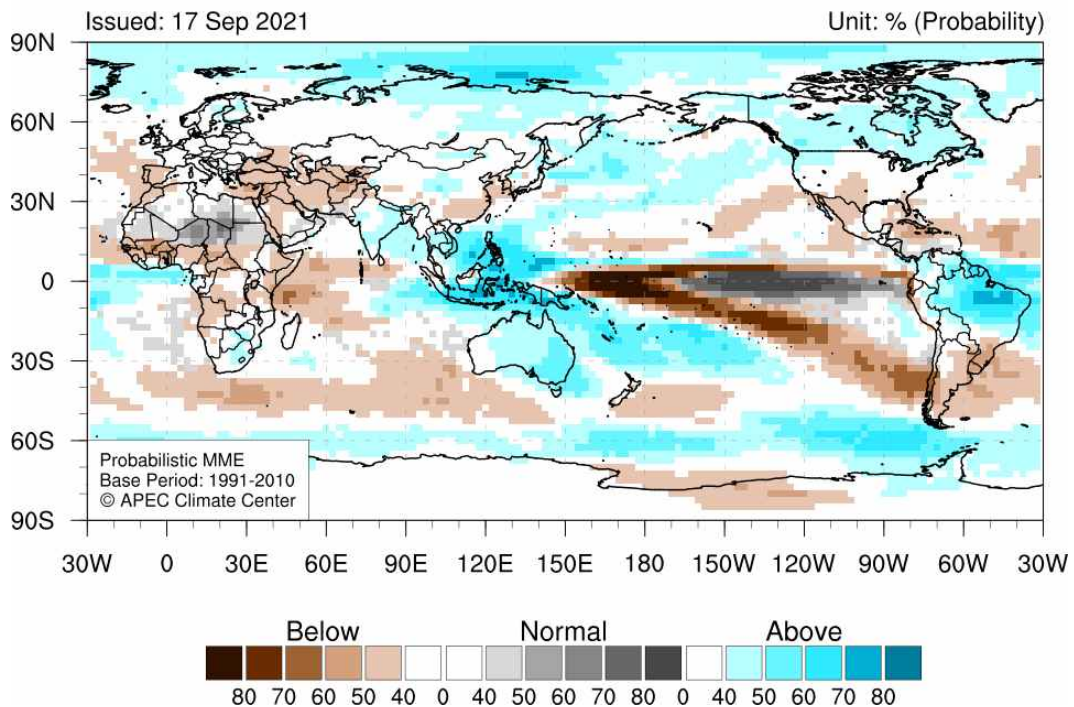
그림 9. (위) 2021년 10월-12월 평균 기온 및 (아래) 강수 평년대비 편차 (평년: 1991-2010).
