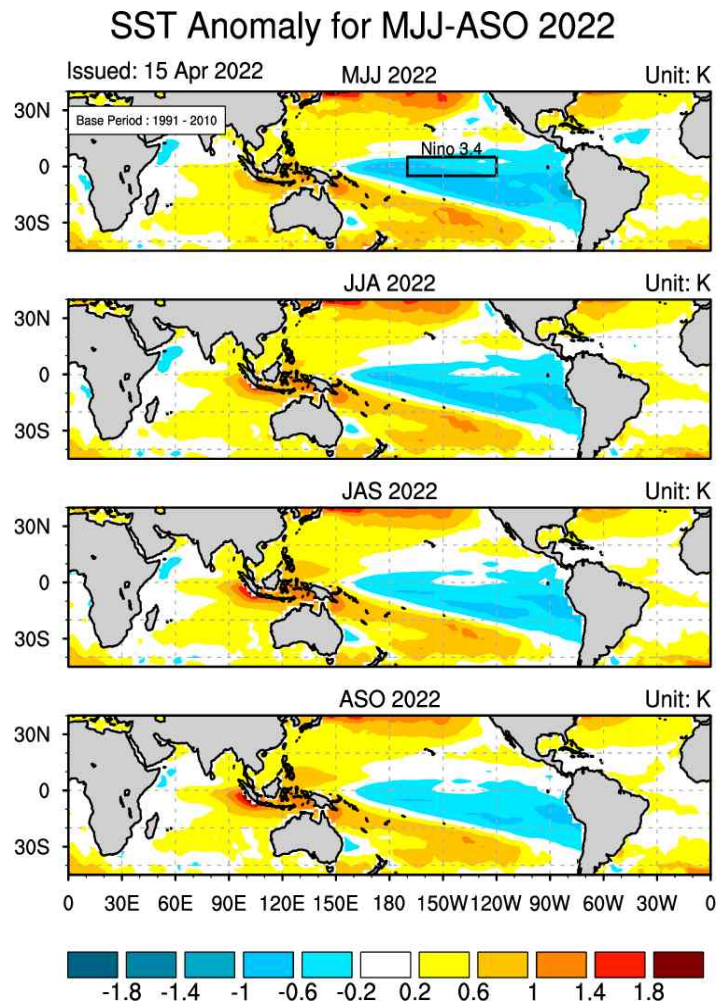
그림 6. 2022년 5월-10월 해수면온도 평년대비 편차(평년: 1991-2010).
