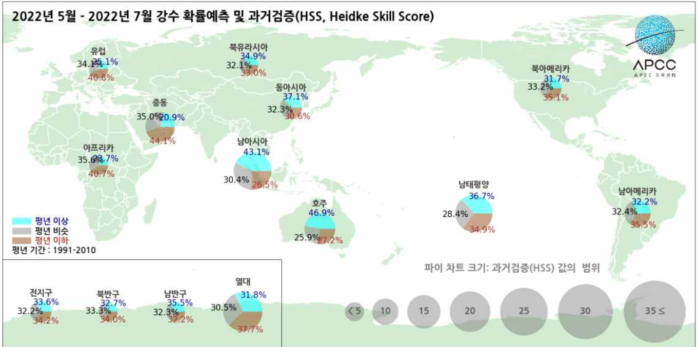
그림 1. 2022년 5월-7월 기온(위)과 강수(아래)의 확률예측 및 과거검증.
