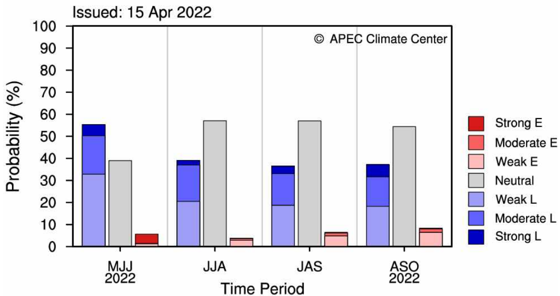
그림 8. 2022년 5월-10월 ENSO 종류 및 강도 확률예측(평년: 1991-2010).
