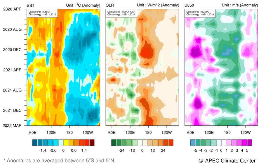
그림 3. 2020년 4월-2022년 3월 해수면온도, 상향장파복사, 850hPa 바람 평년대비 편차의 시간-경도 단면도(평년: 1991-2010).
