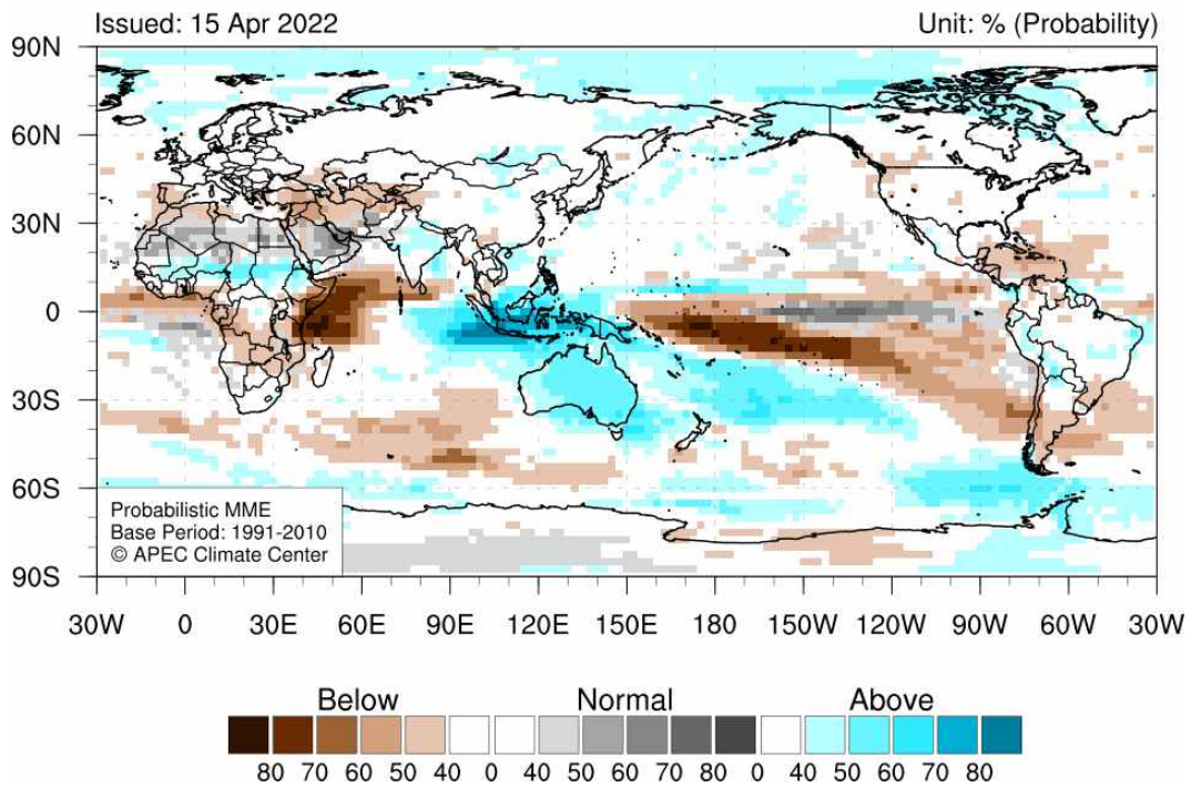
그림 10. 2022년 8월-10월 기온(위)과 강수(아래)의 평년대비 편차(평년: 1991-2010).
