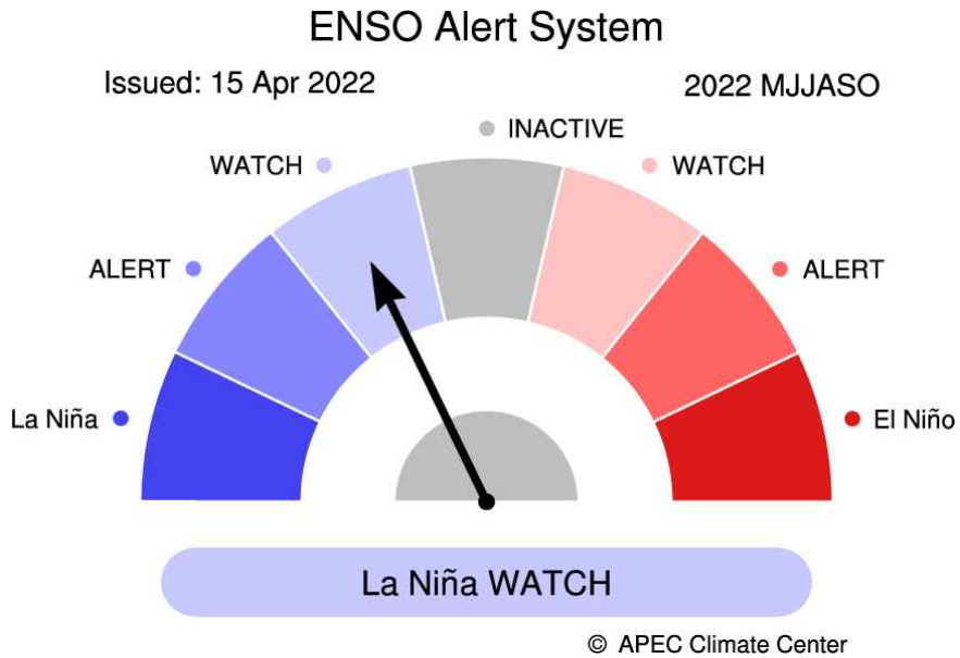
그림 5. 2022년 5월-10월 ENSO 경보(평년: 1991-2010).
