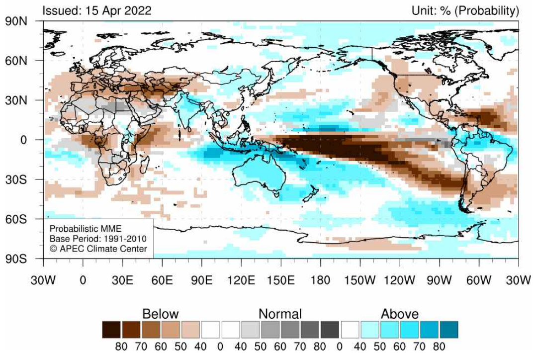
그림 9. 2022년 5월-7월 기온(위)과 강수(아래)의 평년대비 편차(평년: 1991-2010).
