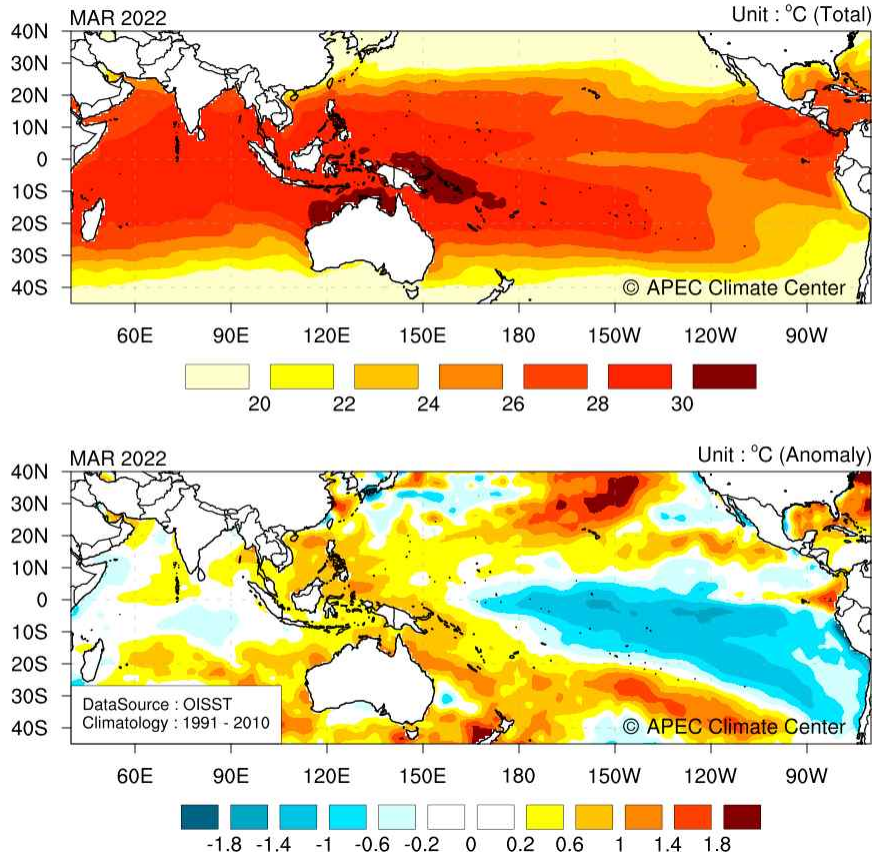
그림 2. 2022년 3월 해수면온도 분포 및 평년대비 편차.
