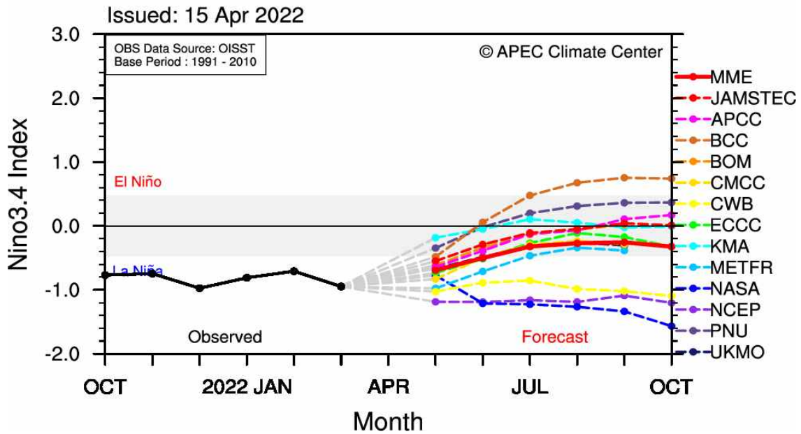
그림 7. 2022년 5월-10월 평년대비 Niño3.4 지수 편차(평년: 1991-2010).
