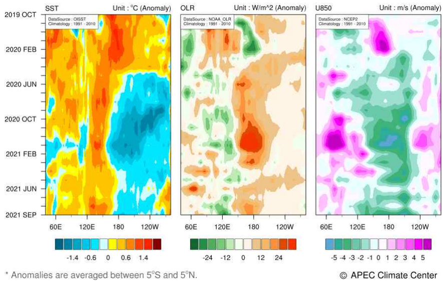
그림 3. 2019년 10월-2021년 9월 해수면온도, 상향장파 복사, 850hPa 바람 평년대비 편차의 시간-경도 단면도 (평년: 1991-2010).
