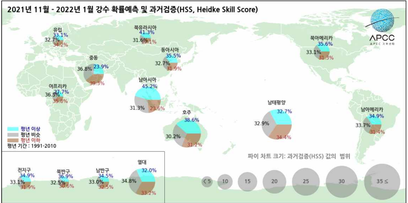
그림 1. (위) 2021년 11월-2022년 1월 평균 기온 및 (아래) 강수 확률예측 및 과거검증.
