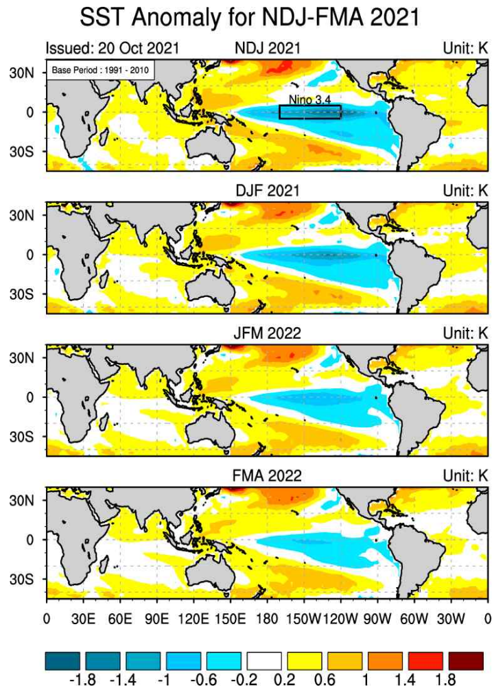
그림 6. 2021년 11월-2022년 4월 평균 해수면온도 평년대비 편차 (평년: 1991-2010).
