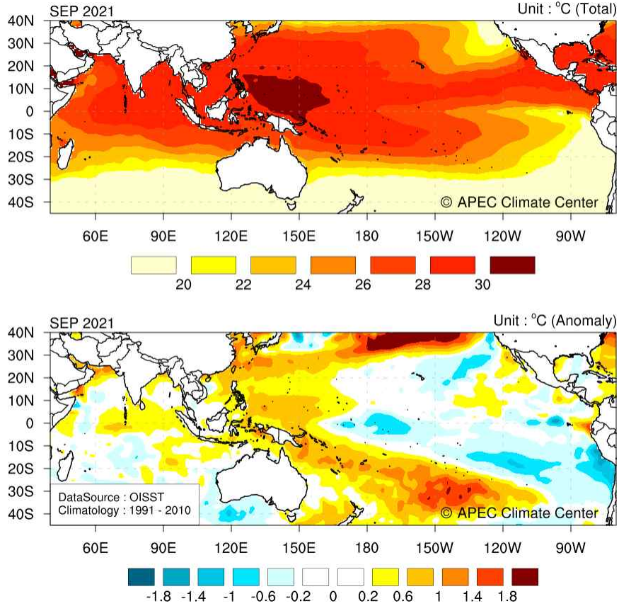
그림 2. 2021년 9월 평균 해수면온도 분포 및 평년대비 편차.
