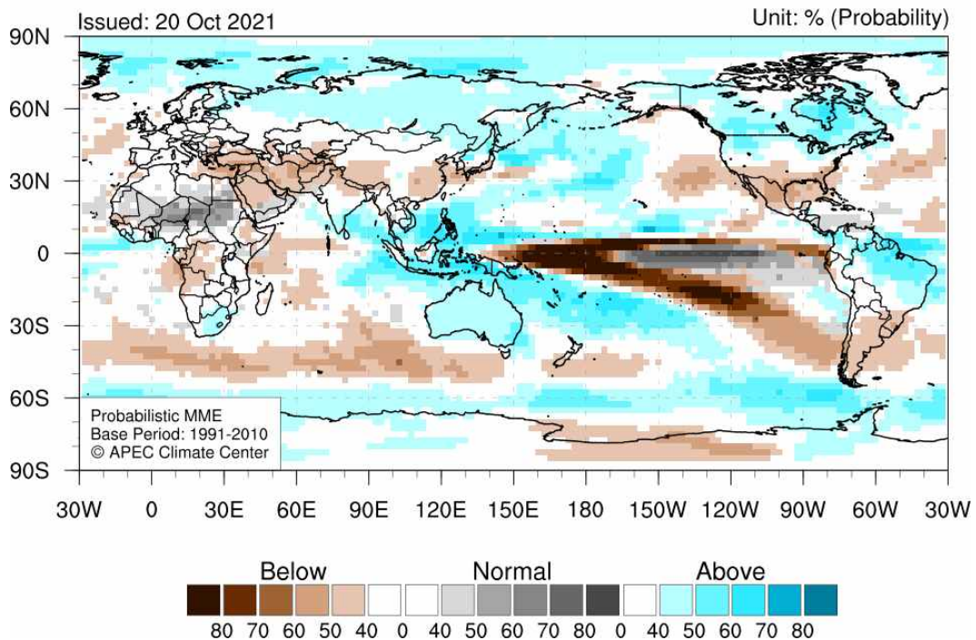
그림 9. (위) 2021년 11월-2022년 1월 평균 기온 및 (아래) 강수 평년대비 편차 (평년: 1991-2010).
