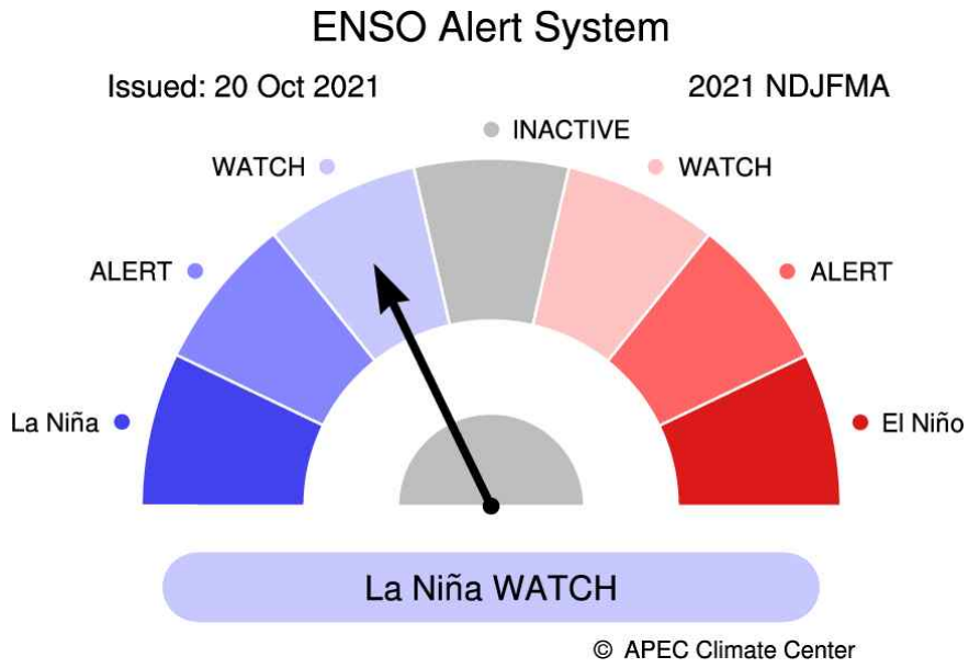
그림 5. 2021년 11월-2022년 4월 ENSO 경보 (평년: 1991-2010).
