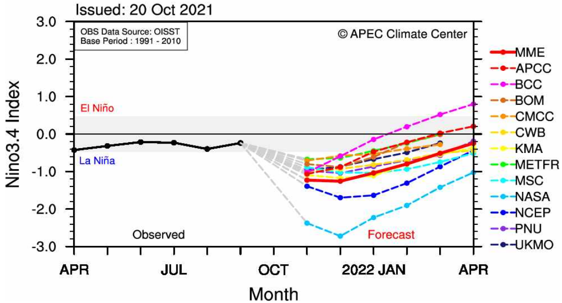
그림 7. 2021년 11월-2022년 4월 평년대비 Niño3.4 지수 편차 (평년: 1991-2010).
