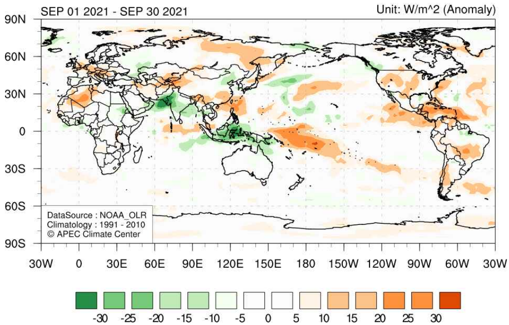
그림 4. (위) 2021년 9월 평균 기온 및 (아래) 상향장파 복사 평년대비 편차 (평년: 1991-2010).
