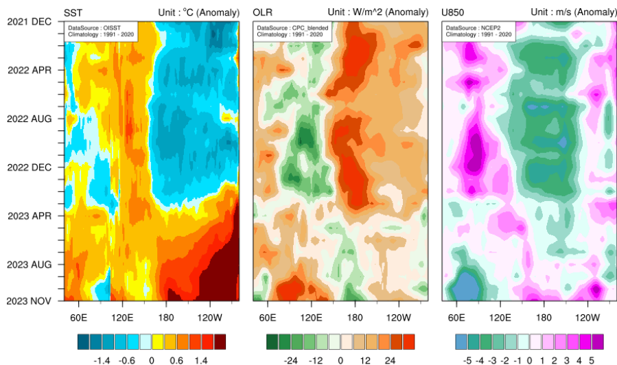
2021년 12월-2023년 11월 해수면온도, 상향장파복사, 850hPa 바람 평년 대비 편차의 시간-경도 단면도(평년: 1991-2020)
